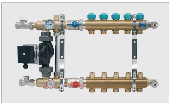
Распределитель для п.о. - серия 73A
