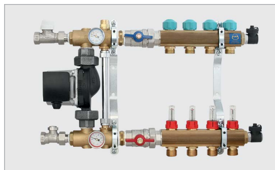
Распределитель для п.о. - серия 77A
